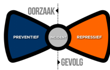
Figuur 12: Vlinderdasmodel
